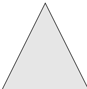
trójkąt (wymiar 2)
