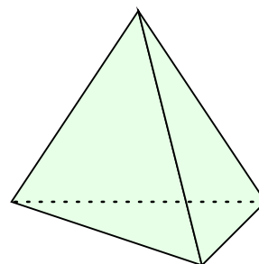
czworościan (wymiar 3)
