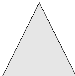
trójkąt (wymiar 2)
